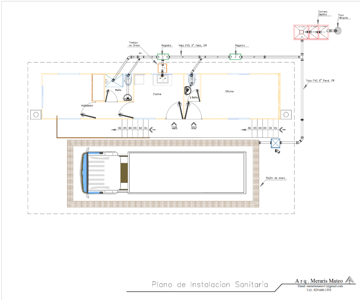
Figura 4: Plano de instalación Sanitaria
