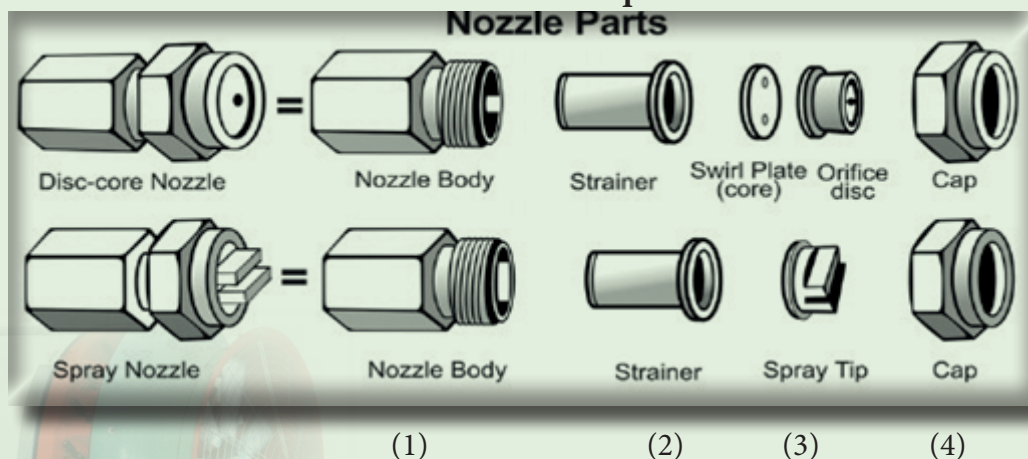
Figura 8-1 Partes de la boquilla. La mayoría de las boquillas se componen de cuatro partes: (1) el cuerpo de la boquilla, (2) la (pantalla) o colador, (3) la punta y (4) la tapa.
