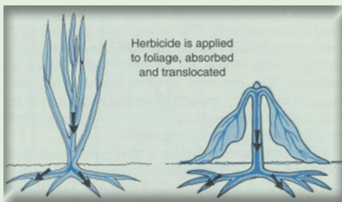
Figura 7-9: Acción de un herbicida selectivo - foliar y sistémico.
