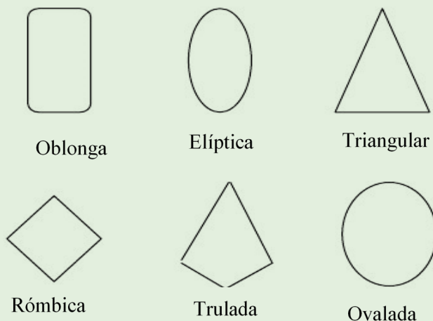
Figura 7-5: ejemplos de formas de una hoja.
