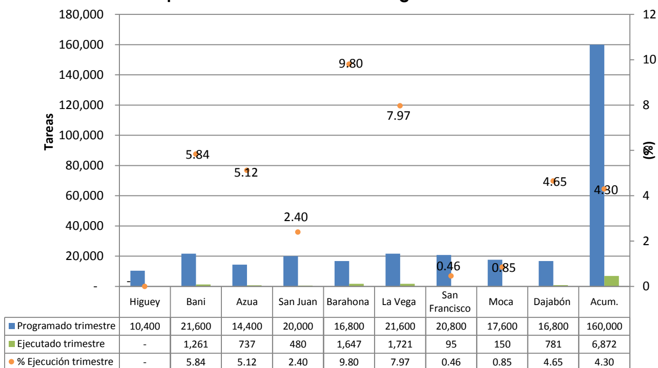
Grafico No. 16 - Comportamiento Mecanización Agrícola
