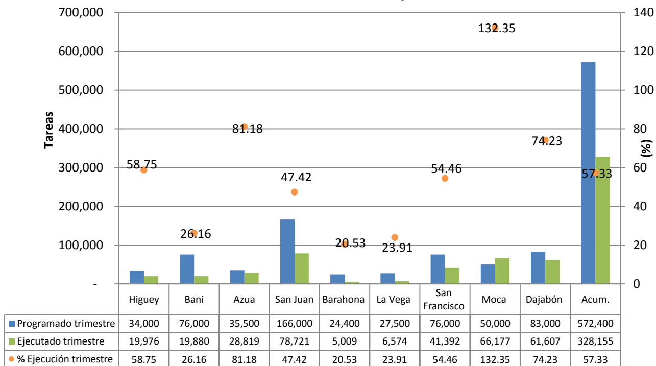
Grafico No. 17 - Comportamiento Mecanización Agrícola
